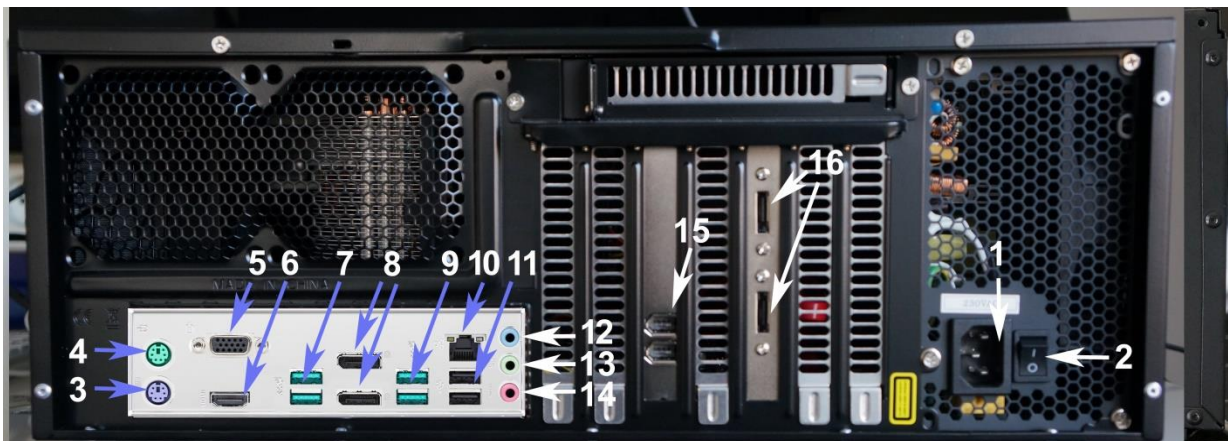
Rückansicht Casablanca 4 SAPHIR 2
